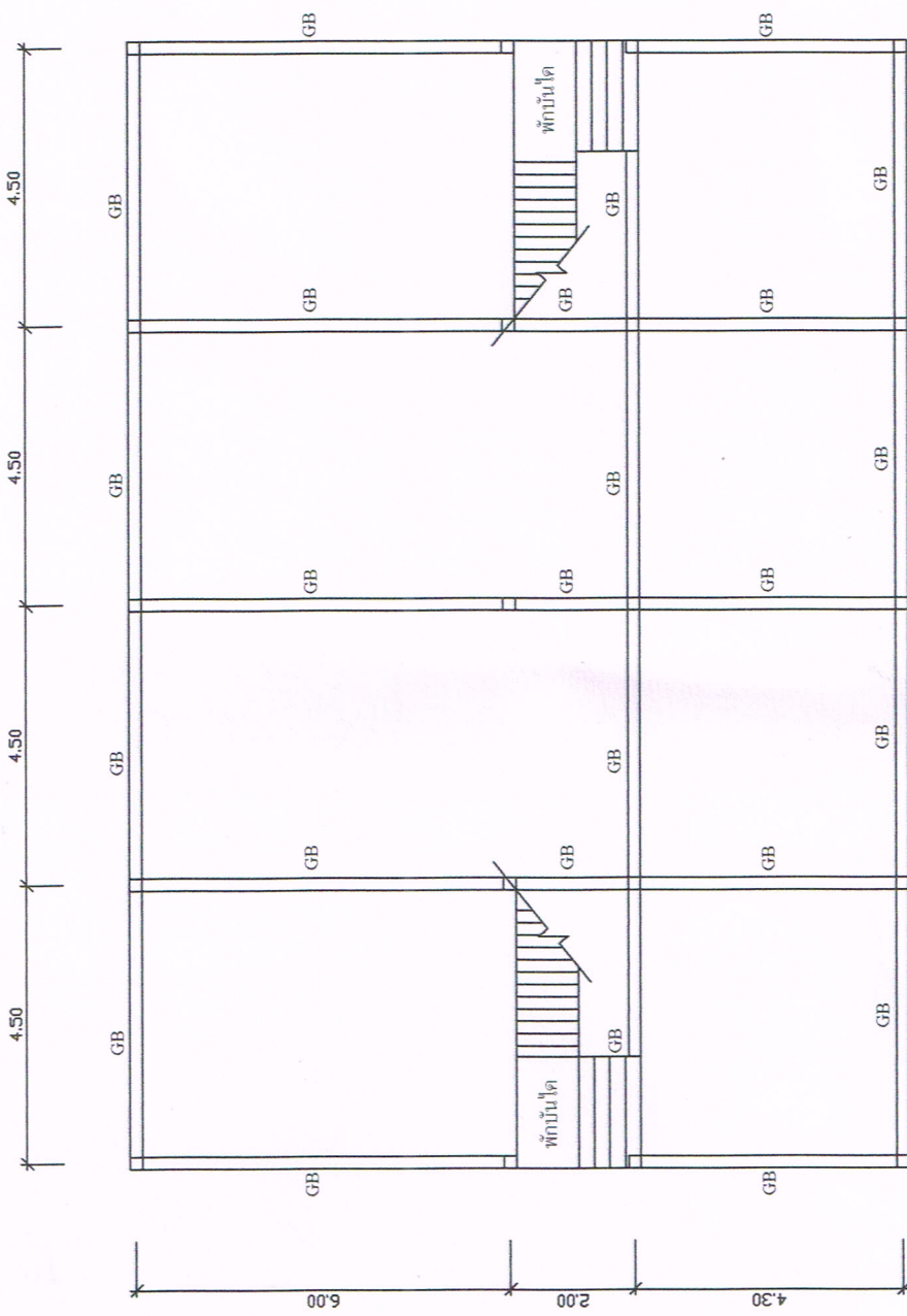
แปลนคานาคอนกรีตโครงการพัฒนา ปรับปรุง ซ่อมแซม อาคารห้องสมุด 1:125
